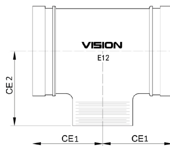
E12 | 内螺纹支口
