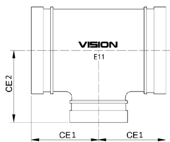
E11 | 沟槽支口
